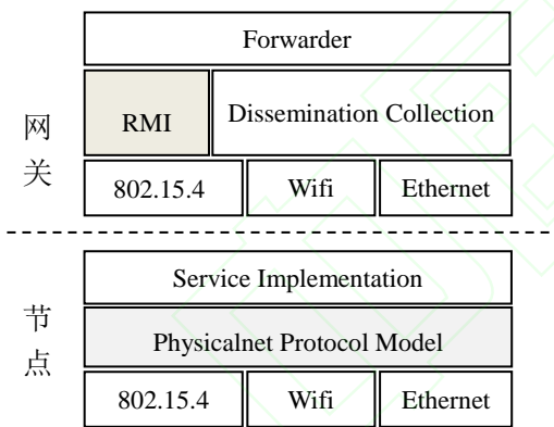
图 3 Physicalnet 物理实体服务的实现架构
