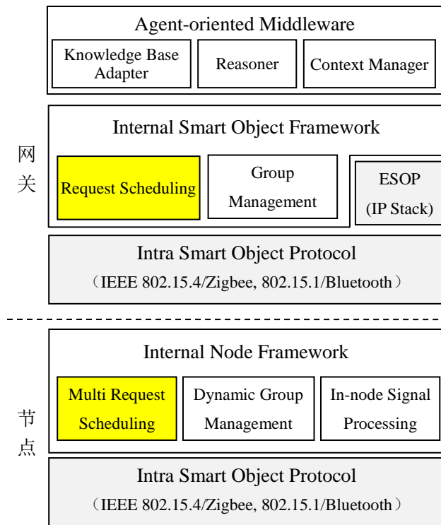
图 4 Agent-oriented Smart Object 的实现架构
